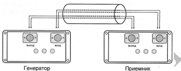
Рис. 5. Измерение переходного затухания на дальнем конце с использованием двух приборов Дельта-ПРО DSL (режим «АЧХ+»).
