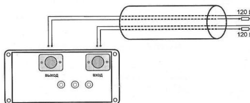
Рис. 3. Измерение переходного затухания на ближнем конце.
