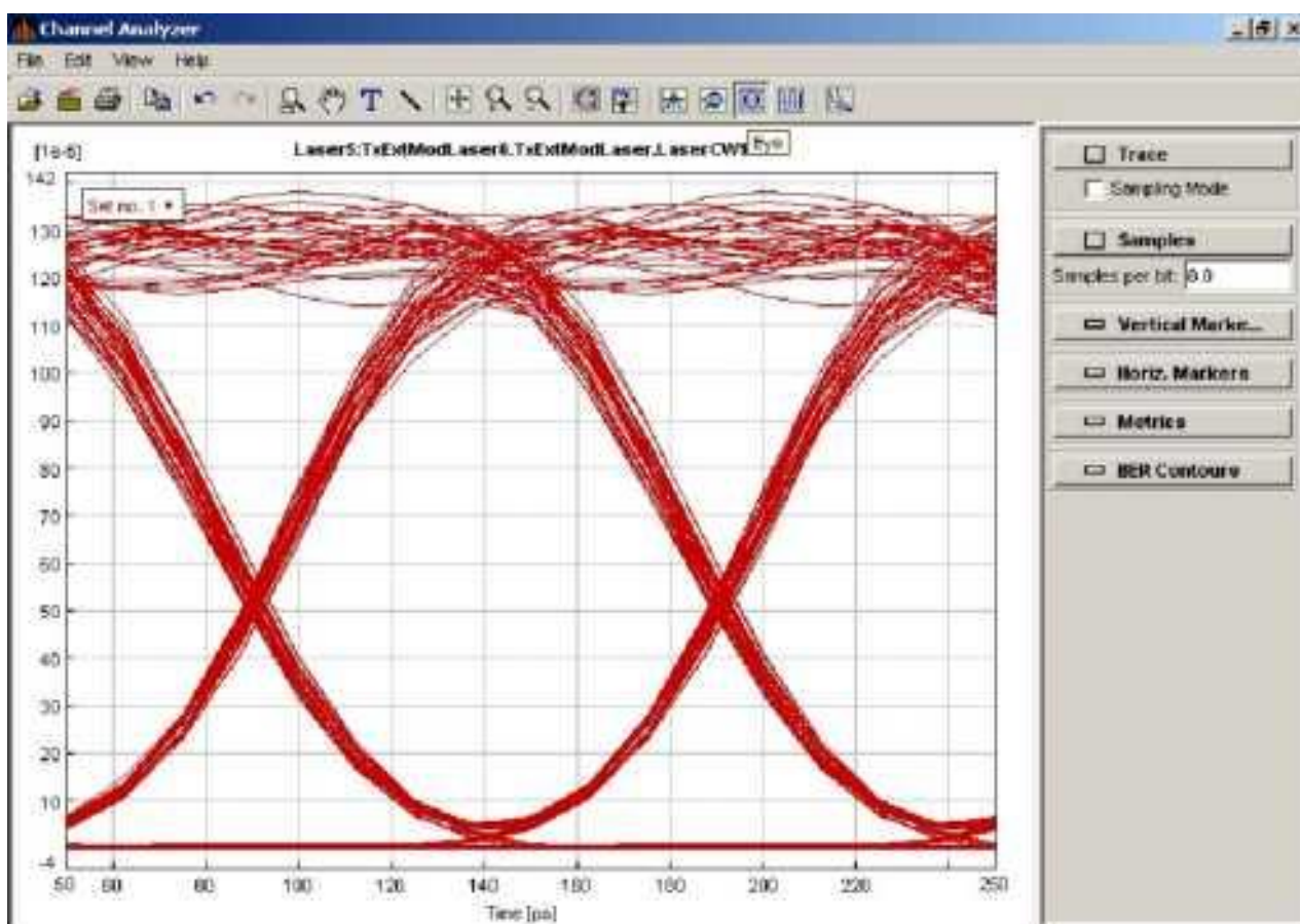
Рисунок 6.1. Глаз – диаграмма, полученная с помощью анализатора канала.
