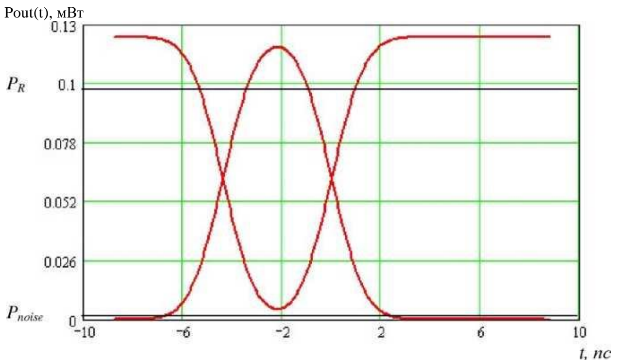
Рисунок 6.2. Пример построения глаз - диаграммы.
