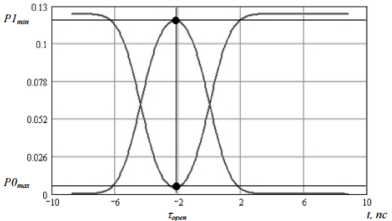
Рисунок 7.2. К оценке параметров распределений состояний «1» и «0».
