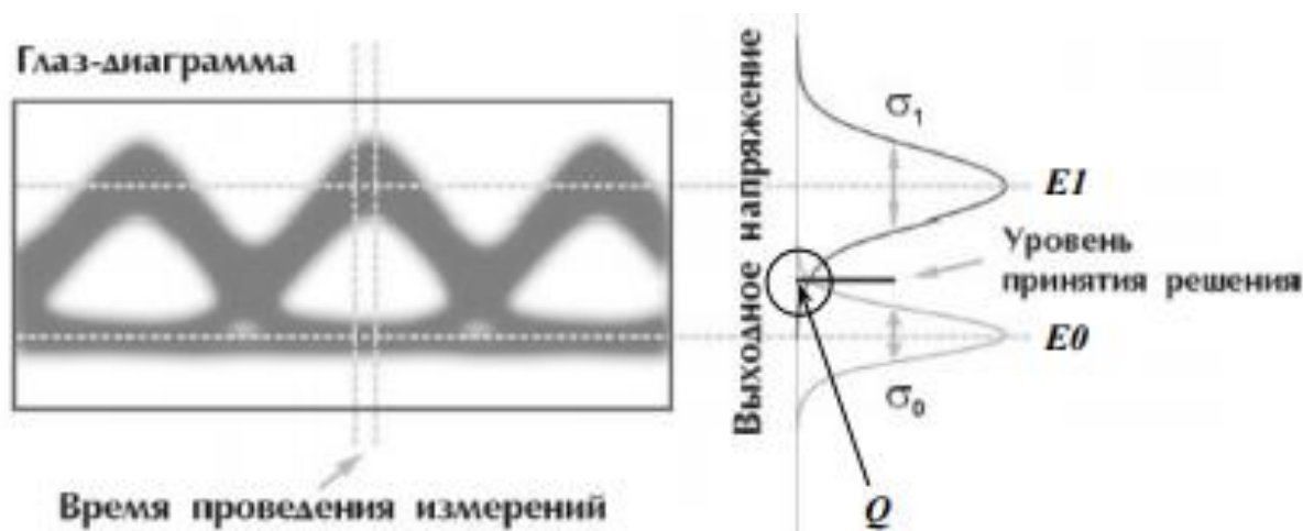
Рисунок 7.1. К оценке Q -фактора.
