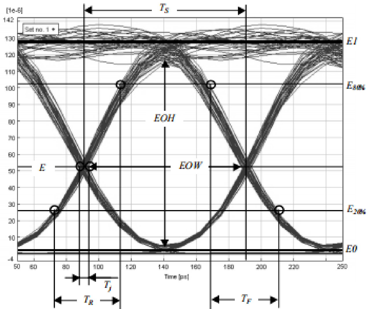
Рисунок 4. Измерение параметров во временной области.
