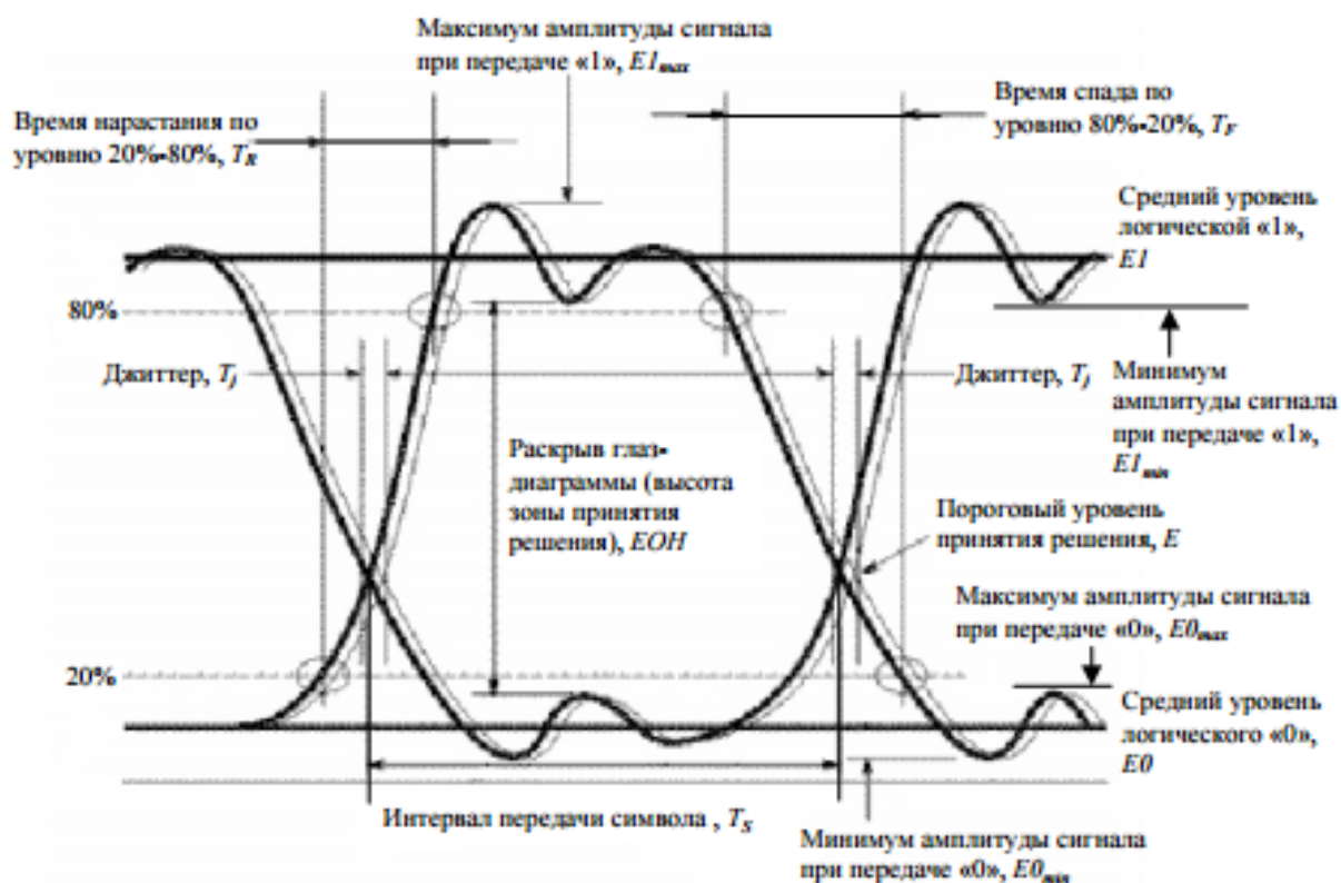
Рисунок 2. Идентификация глаз – диаграммы.
