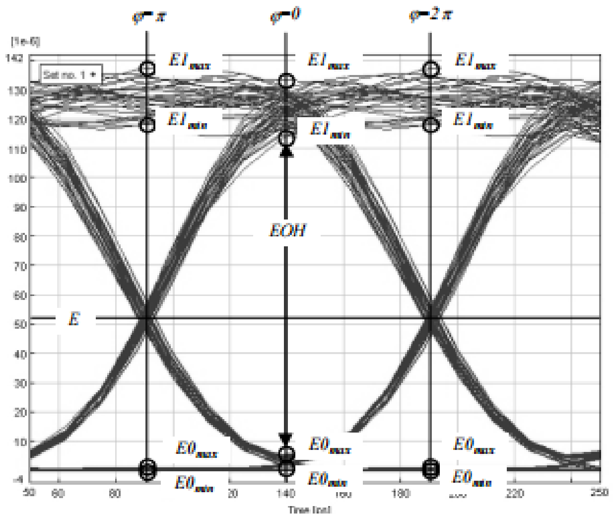
Рисунок 3. Измерение энергетических параметров.
