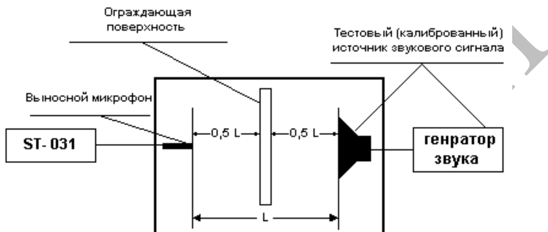
Рисунок 3.1 - Вариант оценки звукоизоляции ограждающей перегородки
