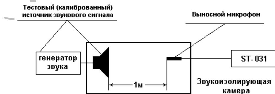
Рисунок 2.1 Схема калибровки индикаторов уровня звукового сигнала прибора ST-031
