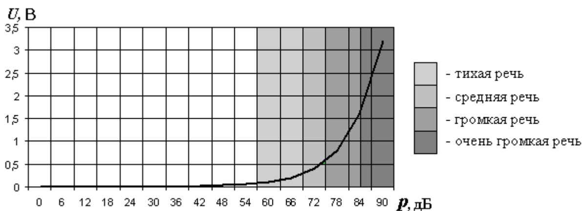
Рисунок 1.1 Перевод уровней акустического сигнала в напряжение.
